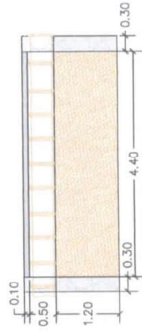
CORTE A – A Escala 1 – 150
